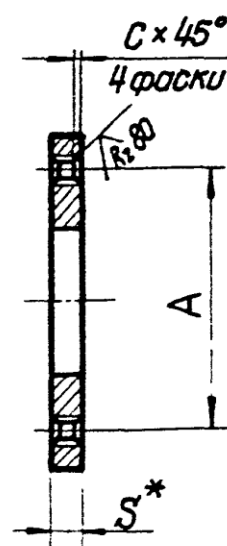
Тип 2 Для дет. 1 (черт. 3)
