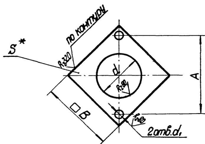
Тип 2 Для дет. 1 (черт. 3)
