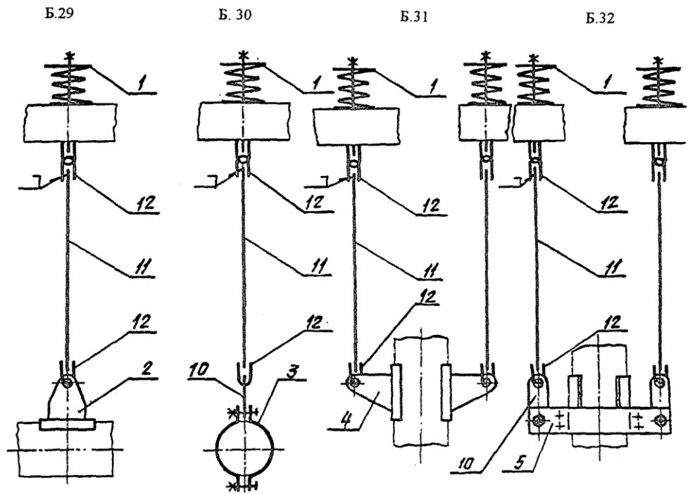
Б.8 Подвески приварные и хомутовые с опорными пружинными блоками. № рисунка
