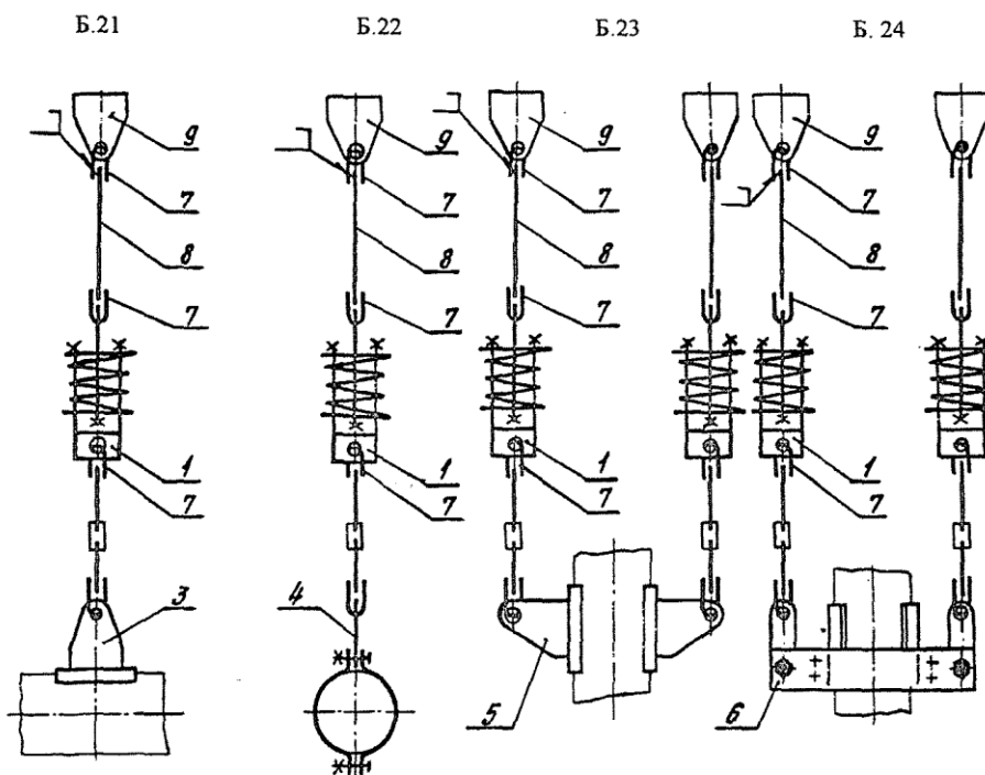
Б.6 Подвески приварные и хомутовые с пружинными блоками № рисунка
