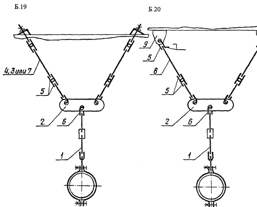
Б.5 Подвески жесткие с траверсой для горизонтальных трубопроводов. № рисунка
