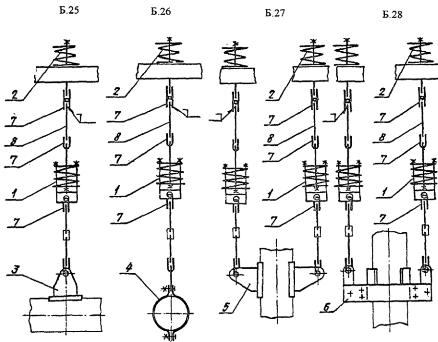
Б.7 Подвески с пружинными блоками и пружинами на перекрытии. № рисунка
