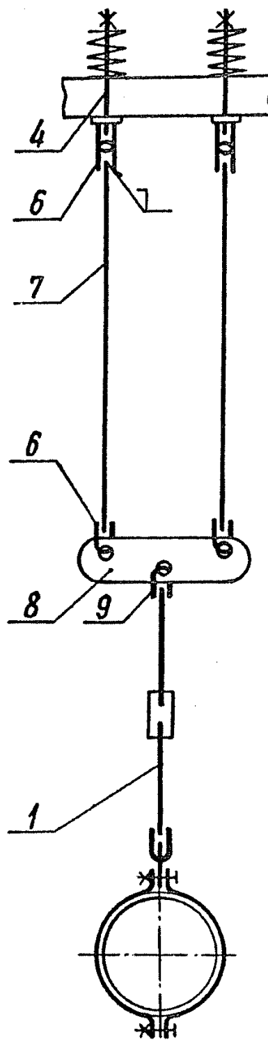
Б 13 Подвески пружинные с траверсой № рисунка
